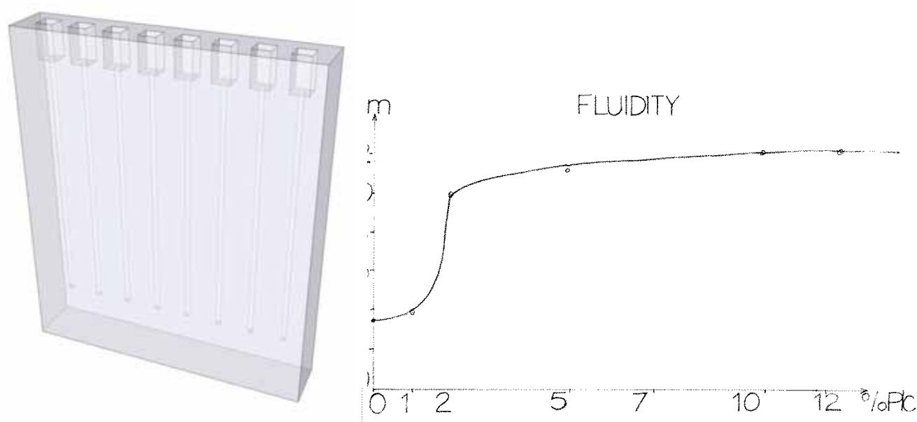
Figure 153 : À gauche, reconstitution du moule utilisé pour les essais de coulabilité d'après la description donnée dans le texte de J. Young (dessin B. Mille) : le moule est à base de sable et mesure 15x20x3 cm (LxHxP). Huit creux de 1x1x2 cm ont été aménagés sur la face supérieure, et un trou de 3 mm de diamètre a été foré au centre de chaque dépression. Une variante différente d'alliage a été coulée dans chaque canal. Il n'est pas signalé que le moule a été préchauffé, la température de coulée est la même pour tous les alliages (1250° C).
