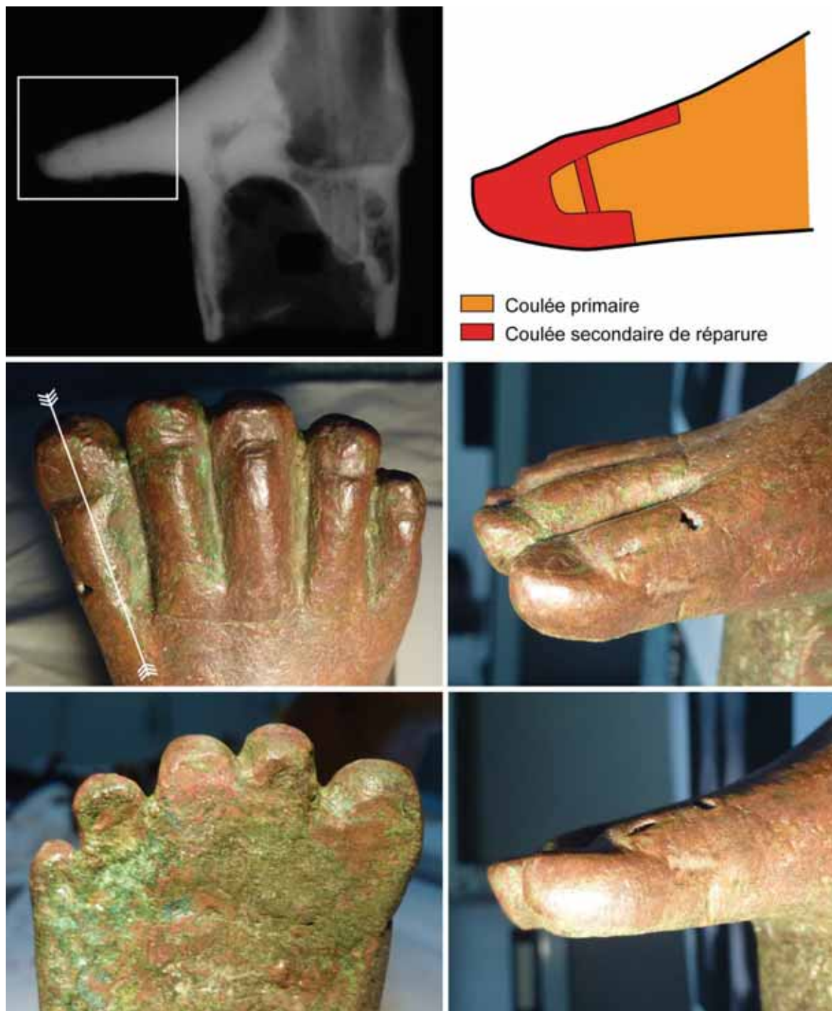
Figure 95 : détails photographiques et radiographique de la coulée secondaire de réparation des orteils du pied droit de la statue de prêtre (E7692). Une coupe longitudinale du gros orteil est présentée comme schéma d'interprétation. La coulée secondaire est visible aussi bien sur la radiographie qu'à la surface du pied. En revanche, le forage de la coulée primaire est une proposition d'explication du mode d'assemblage: l'intrication de la coulée secondaire dans la coulée primaire permettrait le maintien en position de la réparation ( interlock joining ).
