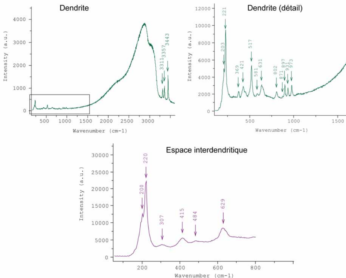
Figure 43 : analyse par microspectrométrie Raman de la rouelle. Le spectre Raman vert a été obtenu sur le composé de couleur verte présent dans les dendrites, le spectre violet est issu du composé rouge de l'espace interdendritique. Pour la localisation précise des deux points d'analyse, cf. Figure 41.
