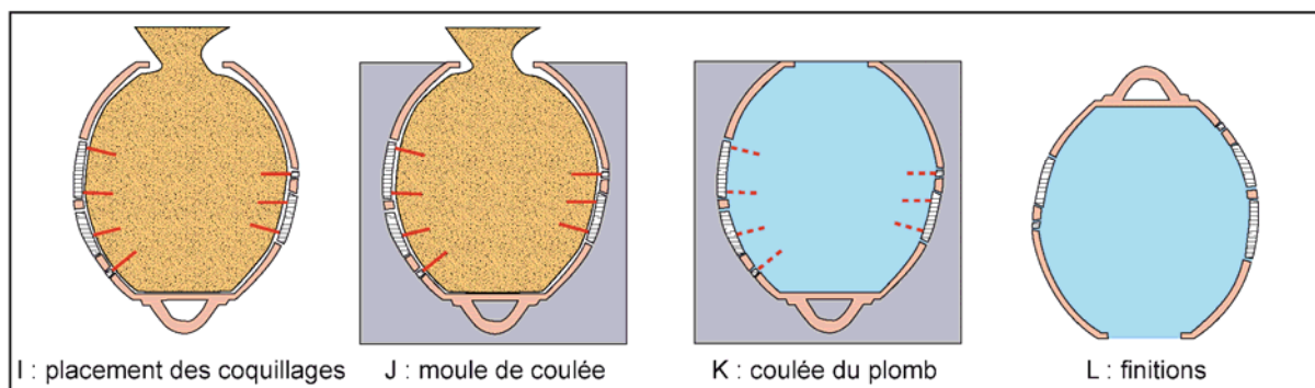
I à L : remplissage par le plomb et incrustation du décor de coquillages (première possibilité)
