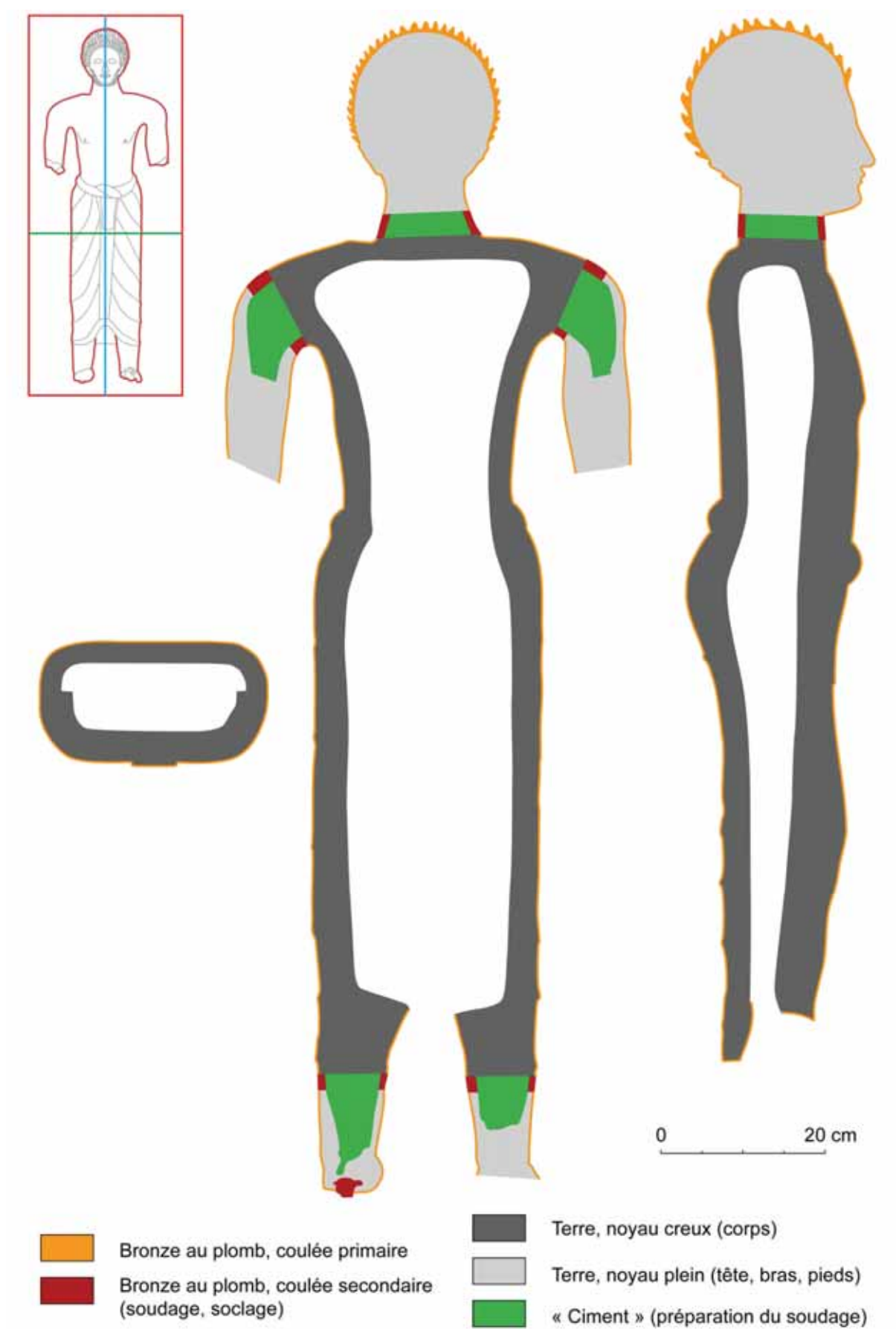
Figure 128 : Hawtar'athat, coupes sagittale, frontale et transversale, schémas déduits des examens radiographiques. En médaillon, localisation des plans de coupe.
