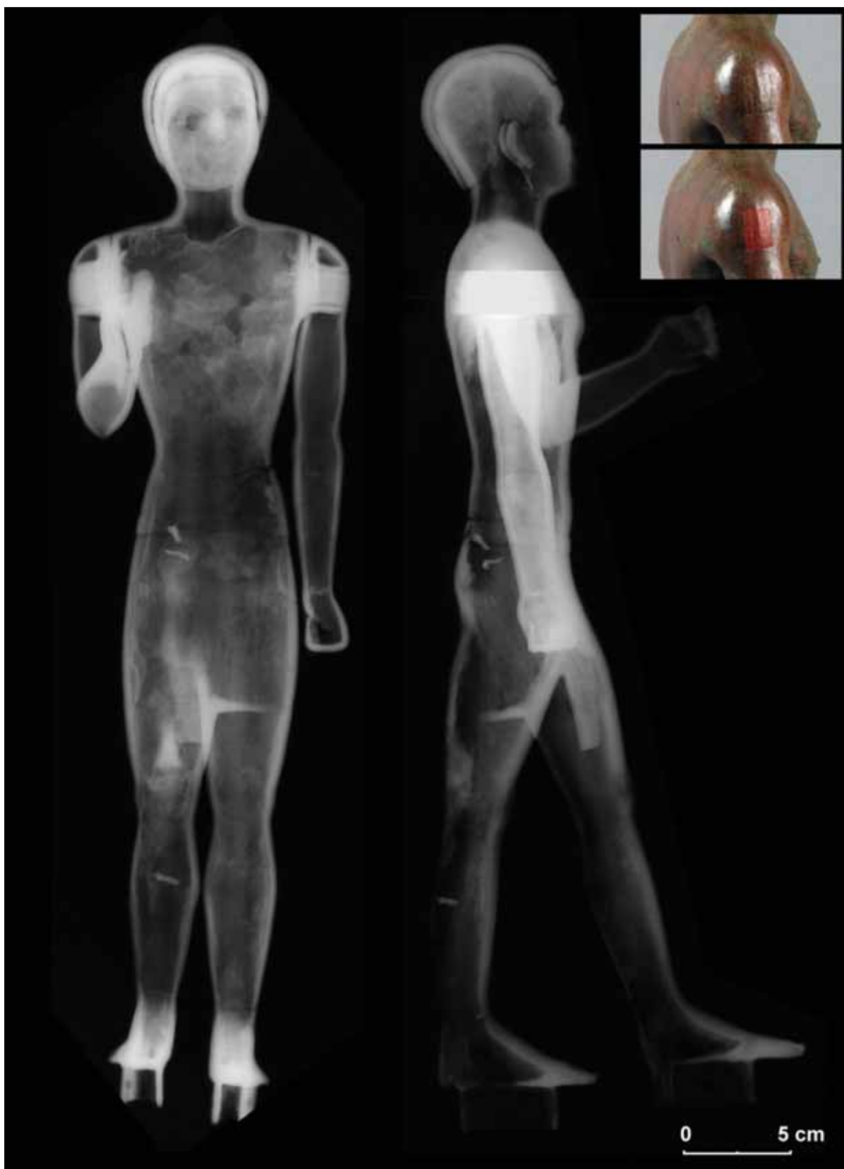
Figure 91 : radiographie X de face et de profil de la statue de Bepeches (n° inv. E7693). En médaillon, photographies de la soudure en boîte du bras droit. La soudure a été effectuée en haut du bras, depuis la face latérale externe, où le métal d'apport affleure directement (figuré par une surimpression rouge sur l'image du bas).
