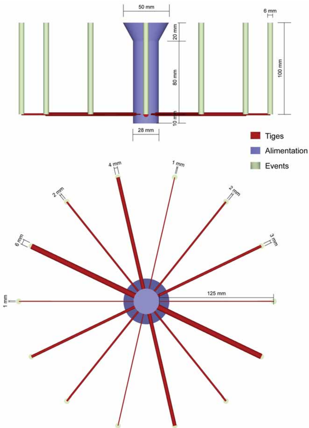
Figure 168 : modèle 3D du test de coulabilité "en araignée", vue de face et vue de dessous, échelle ½.
