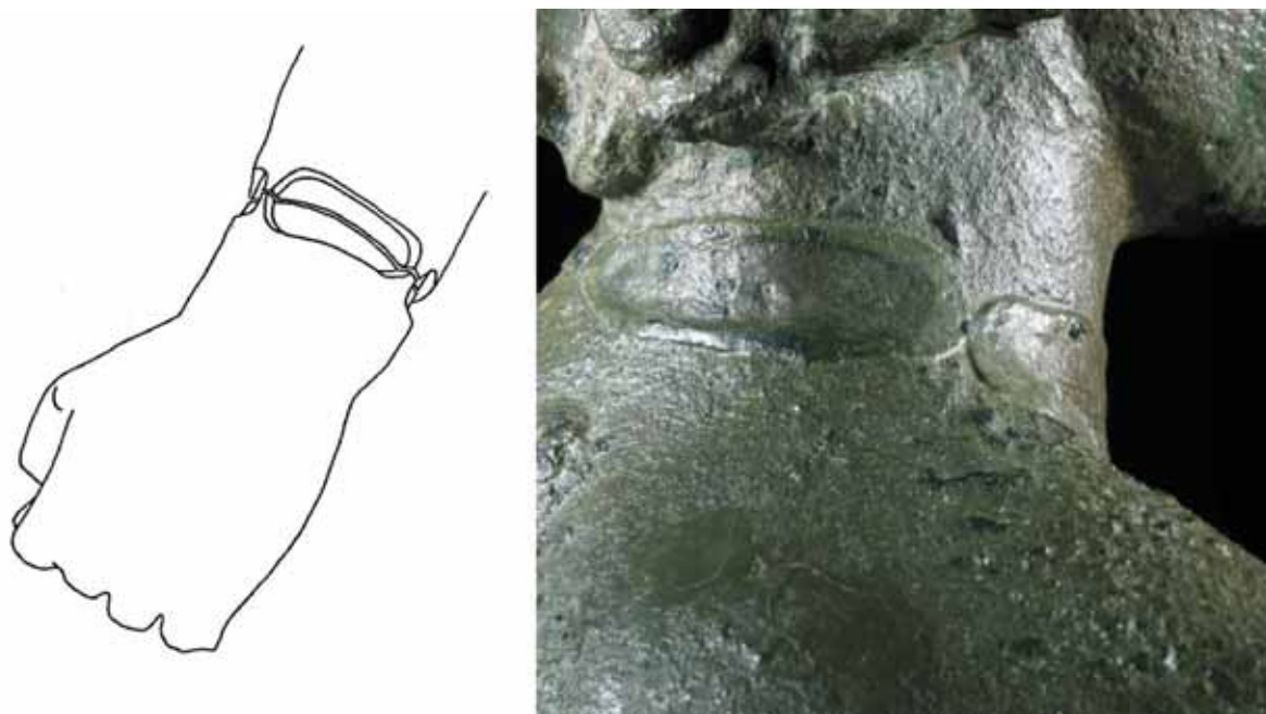
Figure 116 : à gauche : reconstitution schématique de la préparation de la soudure en cuvettes de la main gauche de la statue A de Riace, ce type de cuvette est dit « non traversant » ; à droite : détail de la soudure en cuvettes de la tête de l'éphèbe d'Agde, h. 1,40 m, n°inv. 839, I er s. ap. J.C., musée d'Agde ; la corrosion différentielle des cuvettes explique qu'elles soient si facilement visibles.
