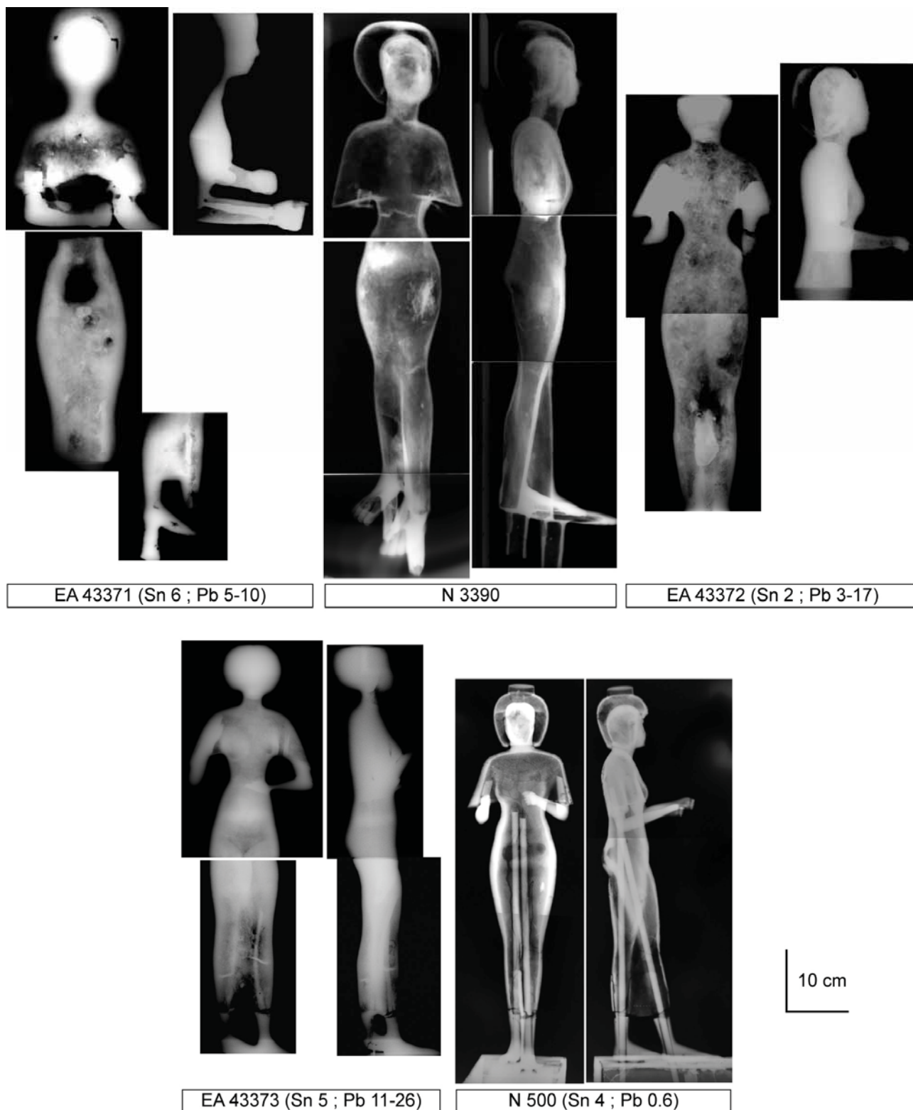
Figure 86 : radiographie X des grandes statues féminines de Karnak. La puissance de l'équipement du laboratoire du British Museum a été insuffisante pour traverser les zones les plus épaisses, il a néanmoins été vérifié que toutes les têtes sont creuses, ce que confirment les radiographies faites au C2RMF sur les deux statues du Louvre. Les teneurs en étain et en plomb sont précisées pour chaque statue, hormis N3390, non analysée. La composition indiquée correspond à la pièce principale (tête+corps+jambes), et non aux pièces assemblées tels que les bras. La variabilité des teneurs en plomb s'explique par la ségrégation du plomb dans la partie basse des statues.
