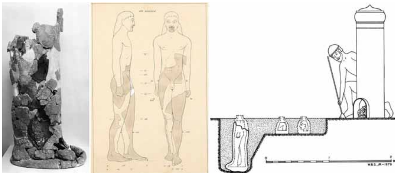
Figure 104 : à gauche, moule d’une statue de kouros découvert dans sa fosse de coulée sur l’Agora d’Athènes, à proximité du temple d’Apollon Patroos, h. 0.75 m, milieu du VI e s. av. J.-C ; au milieu, proposition de reconstitution de la statue d’après le tirage en plâtre des empreintes encore existantes dans les différents fragments de moule ; à droite, reconstitution de la fosse de coulée avec en place les moules des trois pièces à couler (tête, haut du corps, bas du corps).
